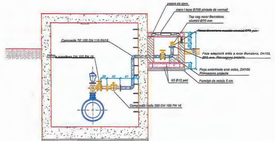
SECCIÓ A - A' ESCALA 1:50
