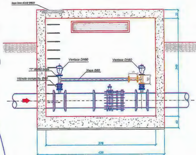
PLANTA ESCALA 1:50
